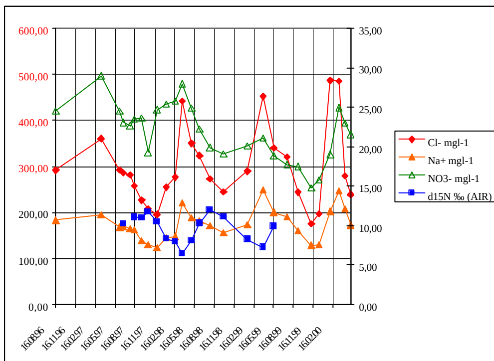
Abb. 7-10: Analyse zur Entwicklung der Brunnenwasserbeschaffenheit ausgewählter Parameter des Referenzbrunnens SB/F68
