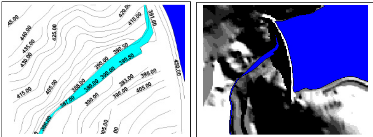
Abb. 52: Aufwändige und generalisierte Höenerfassung morphologischer Strukturen am Beispiel des Stau-mauerfußes der Saidenbachtalsperre
