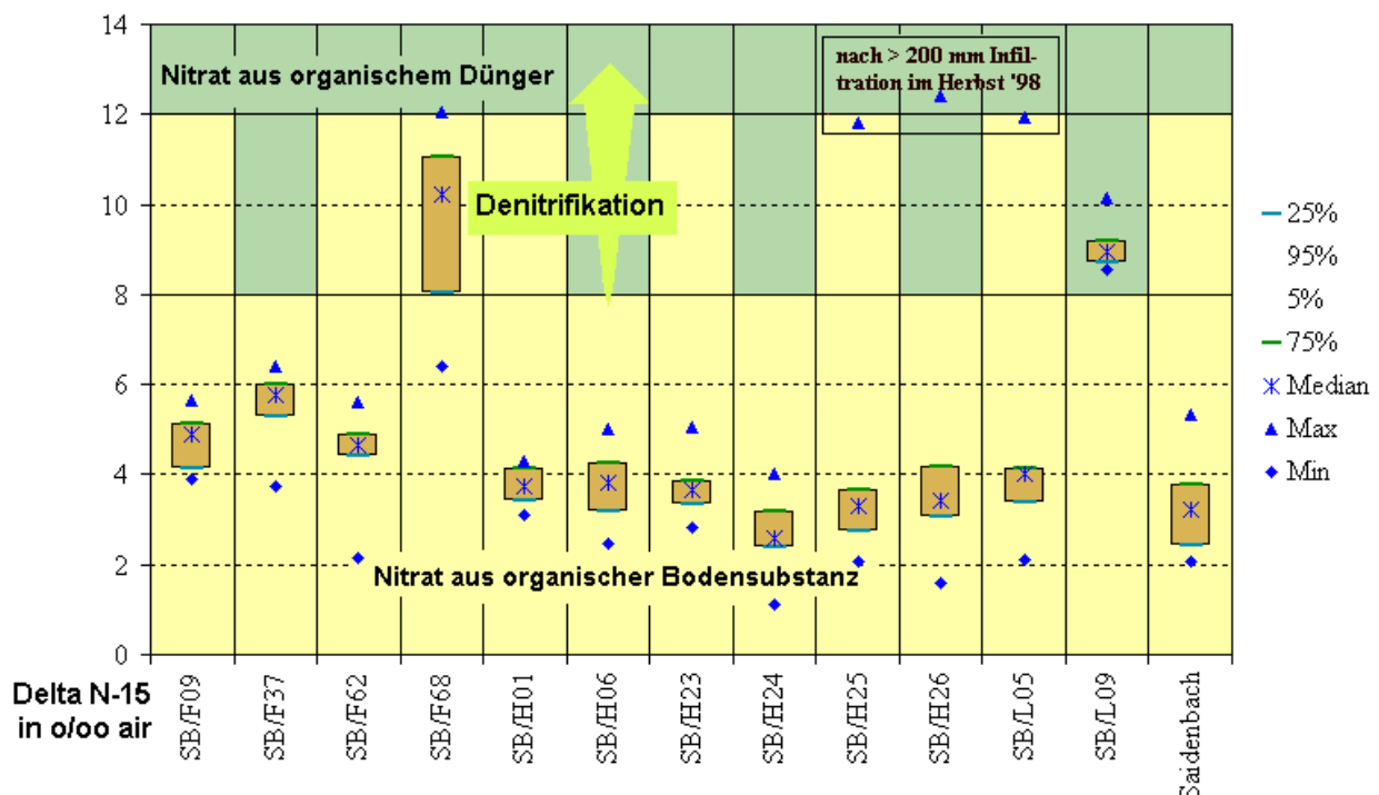
Abb. 7-6: Box-Whisker-Diagramm zur Darstellung der Variabilität der \delta^{15}\text{N} -Gehalte im Brunnenwassernitrat ausgewählter Referenzbrunnen und im Vorfluter Saldenbach
