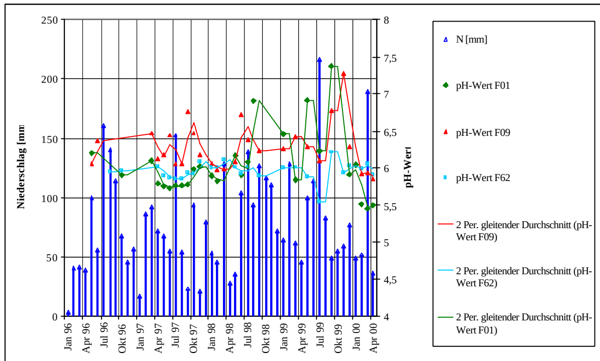
Abb. 6-8: Monatliche Niederschläge und pH-Wert-Verlauf ausgewählter Referenzbrunnen
