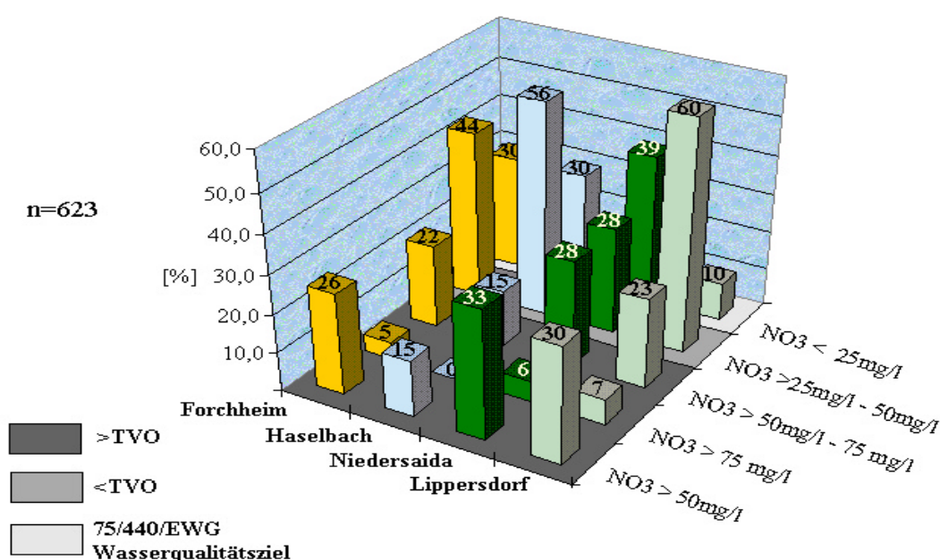
Abb. 65: Prozentuale Verteilung unterschiedlicher Klassifizierungen der Nitratkonzentration in den Gemarkungen der Brunnendörfer aus der Übersichtsbeprobung (Referenzbrunnenzeitreihen als Medianwerte)
