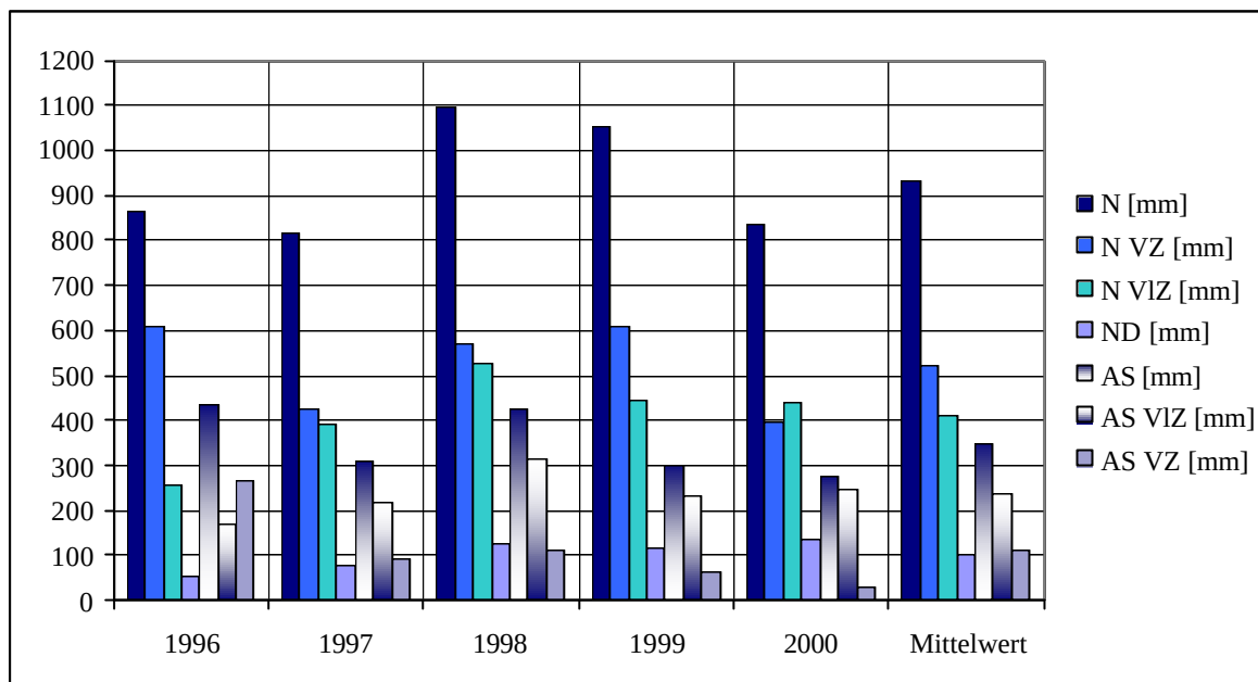
Abb. 7-1: Mit „WRAP“ für Flachbrunneneinzugsgebiete des Untersuchungszeitraums berechnete mittlere Raten des Direktabflusses ( N_D ) sowie der Versickerung ( A_S ) in der Vegetations- (VZ) und vegetationslosen (VIZ) Zeit
