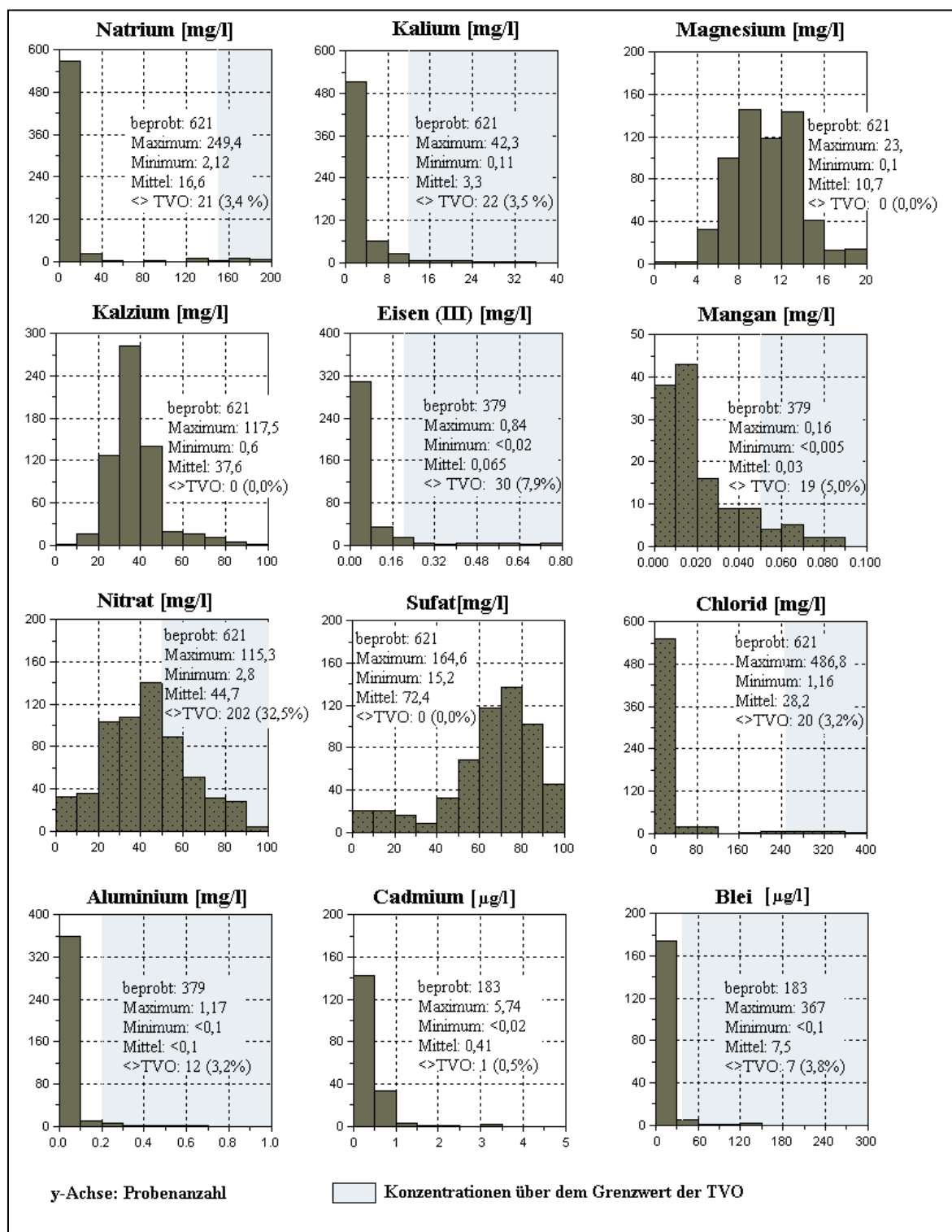
Abb. 6-4: Histogrammdarstellungen und Statistik (Maximum, Minimum, arithmetisches Mittel) zur Häufigkeitsverteilung von ausgewählten Kationen, Anionen und Metallkonzentrationen aus der gesamten Beprobungskampagne (6/1996 bis 12/2000)
