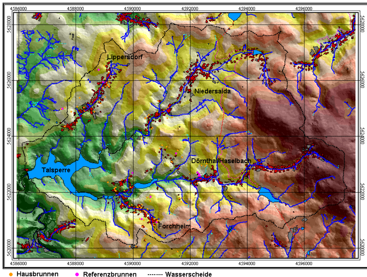
Abb. 1-1: Einzugsgebiet der Saldenbachtalsperre – aus dem Digitalen Geländemodell abgeleitetes Schummernungsmodell mit Höhenschichtung
