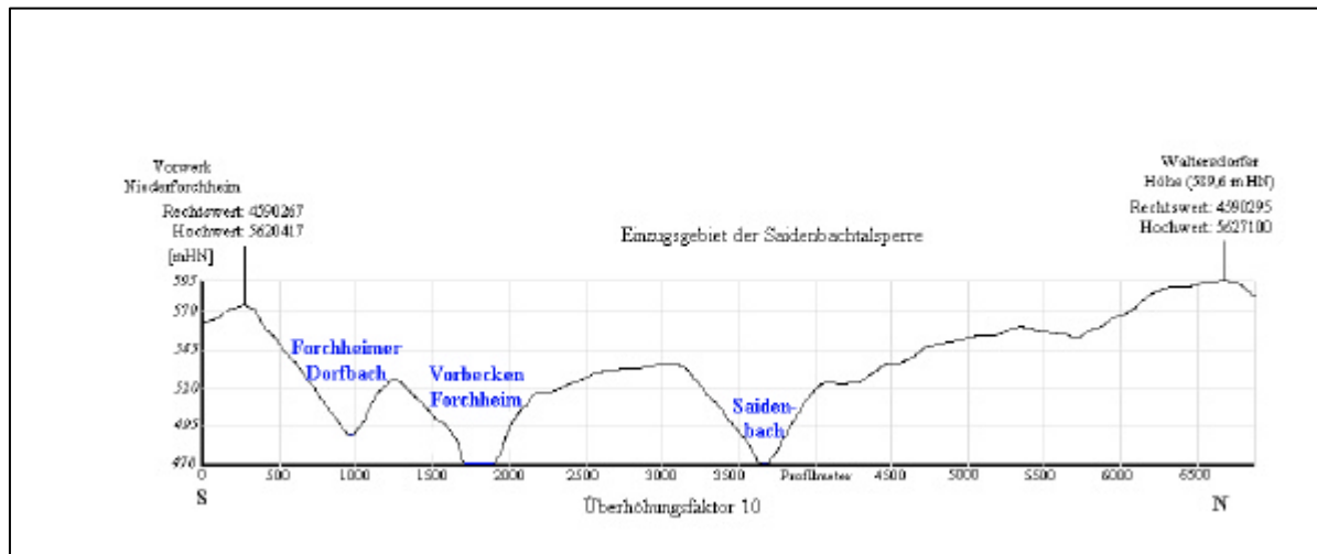
Abb. 5-5: Süd-Nord-Querschnitt durch das Einzugsgebiet der Saidenbachtalsperre auf Grundlage des DGM
