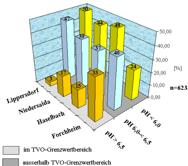
Abb. 6-7 Prozentuale Verteilung unterschiedlicher pH-Wert-Klassifizierungen in den Gemarkungen der Brunnendörfer
