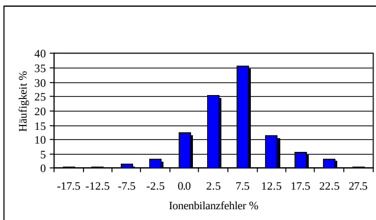
Abb. 62: Prozentuale Häufigkeitsverteilung der Ionenbilanzfehler für 623 Vollanalysen von Hausbrunnenwässern
