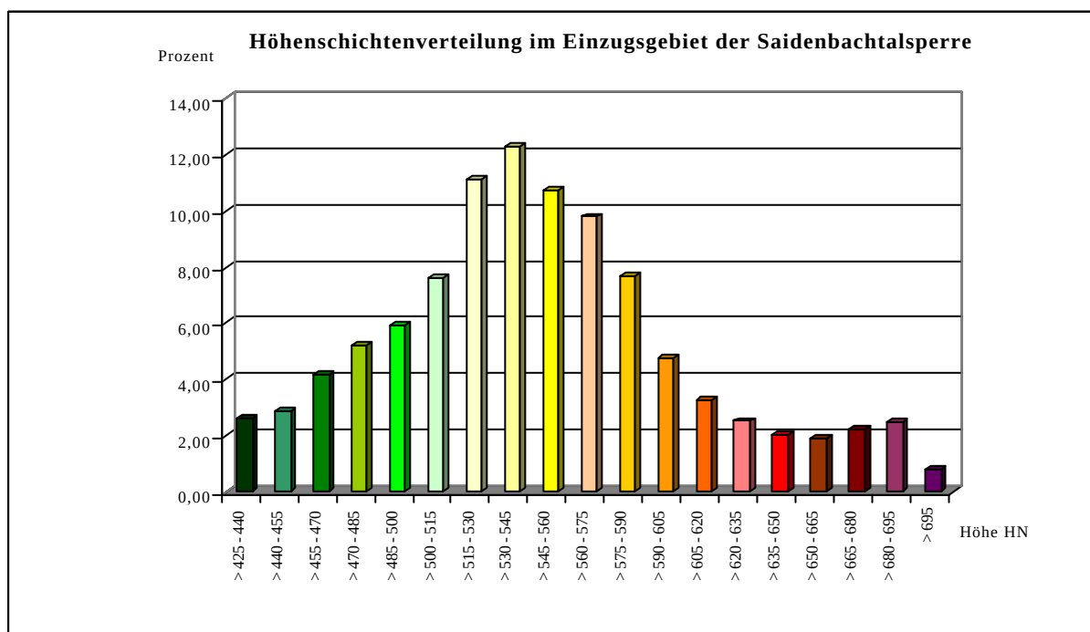
Abb. 5-6: Höhengschichtenverteilung im Einzugsgebiet der Saidenbachtalsperre abgeleitet aus dem DGM
