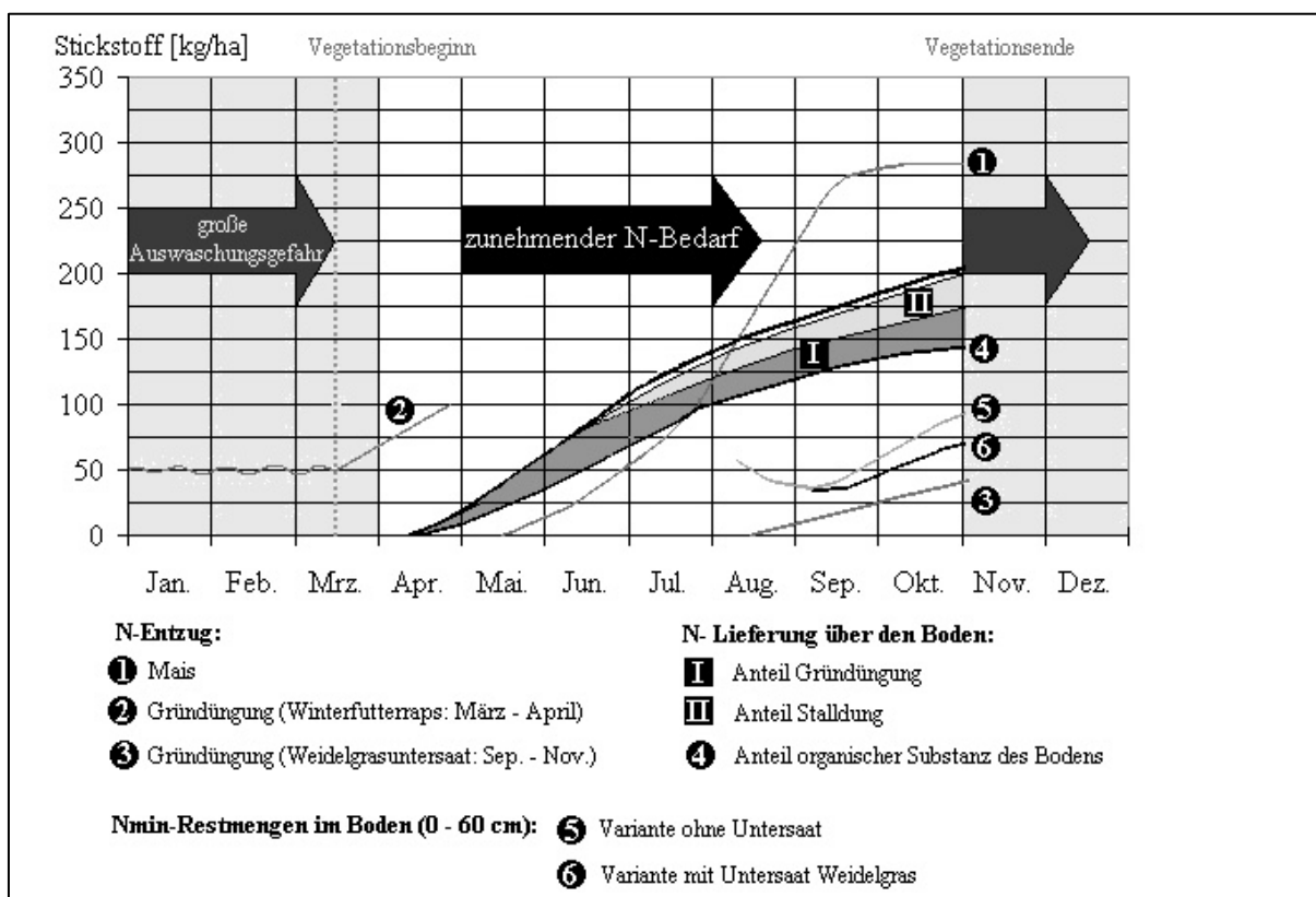
Abb. 6-1: Stickstoffaufnahme von Mais, Winterfutterraps und Weidelgrasuntersaat sowie Stickstoffquellen und mineralisierte Restmengen im Boden (nach MICHALSKI, 2000 verändert)
