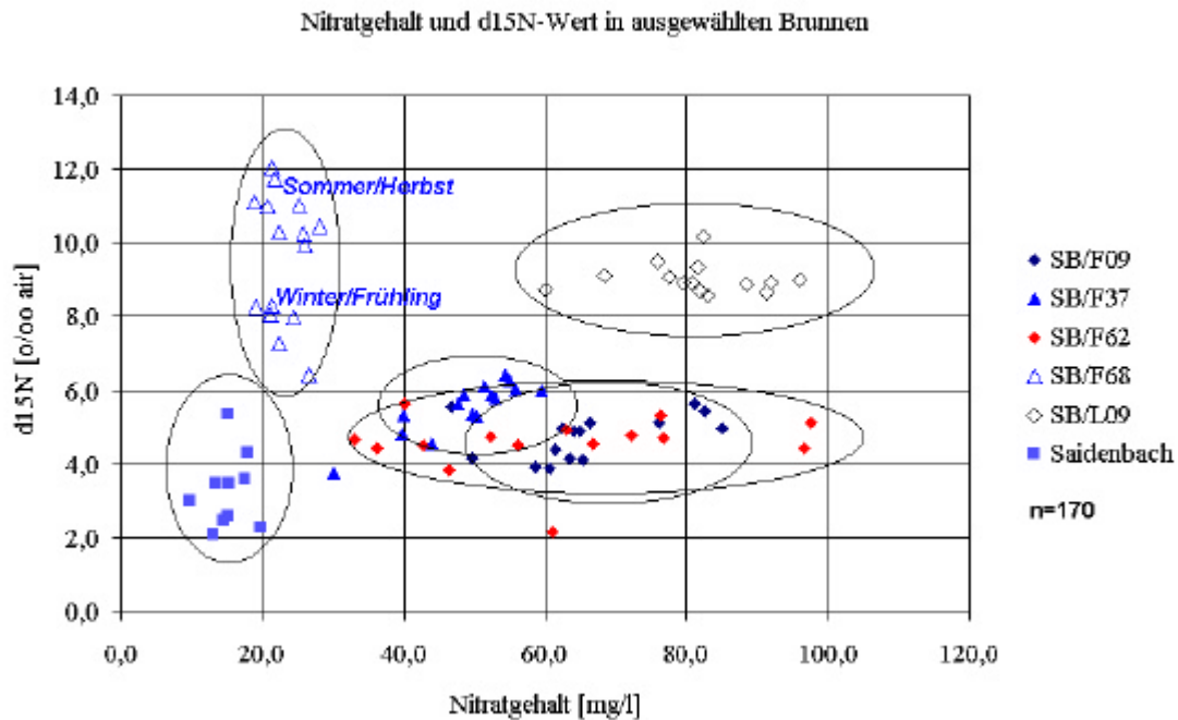
Abb. 7-5: Nitratgehalte und \delta^{15}\text{N} -Werte ausgewählter Referenzbrunnen im Zeitraum zwischen Juni97 bis Mai99
