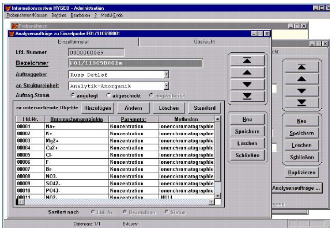
Abb. 2-6: Analysenauftrag in der Datenbank „HYGEO“
